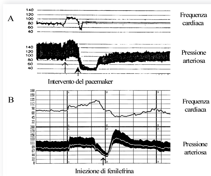
Figura 1. Effetti dell'intervento del pacemaker (A) e della somministrazione di fenilefrina (B) durante la sincope tilt-indotta. Il pacemaker vicaria la bradicardia ma non risulta efficace nell'ostacolare l'ipotensione e quindi nell'abortire la sincope. La fenilefrina determina un rapido incremento della pressione arteriosa capace di abortire la sincope, nonostante un'ulteriore riduzione della frequenza cardiaca.
